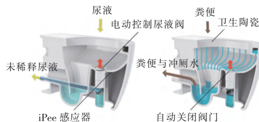
图 2 电控感应粪尿分离厕所
