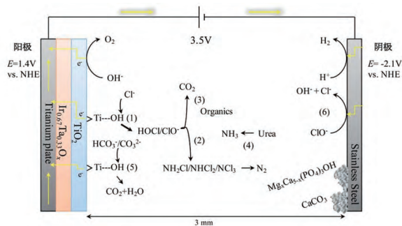
图 12 厕所污水电解处理原理
