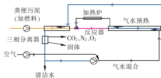
图 7 超临界水氧化技术处理粪便污泥原理
