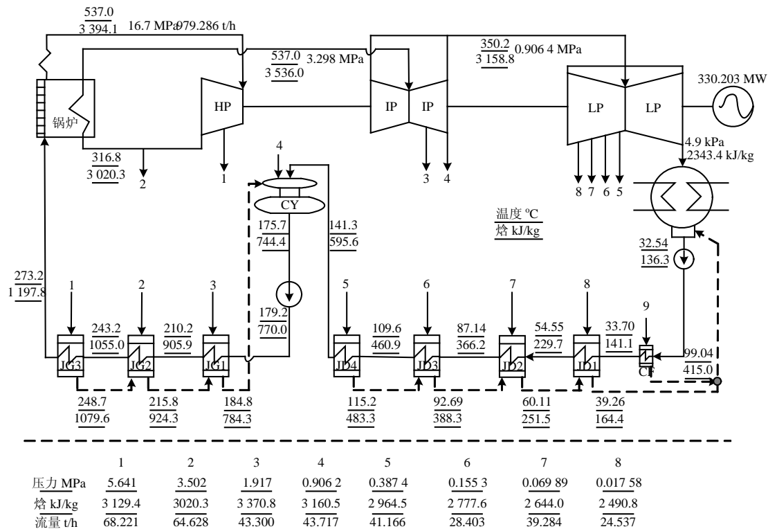
图 2 330 MW 电厂额定负荷热力系统简图
